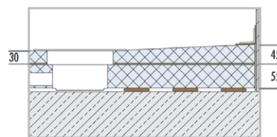
waagerechter Ablauf mit Unterbauelement
