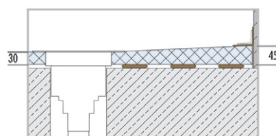
senkrechter Ablauf ohne Unterbauelement
