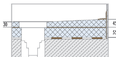
senkrechter Ablauf mit Unterbauelement
