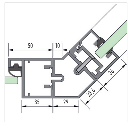
6 Zargenprofil mit Eckprofil 135° + Wandprofil
