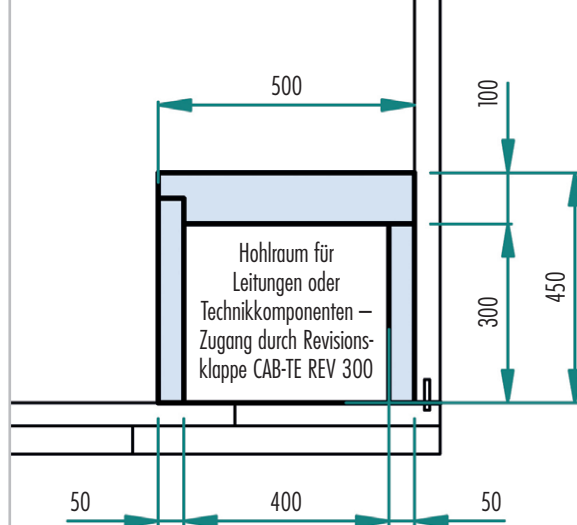
Maße Sitzbank
