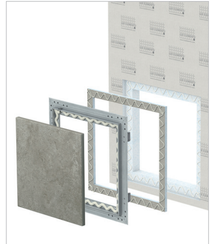
Anwendung bei Naturstein: ohne Frontplatte / Füllstücke unter Rahmen
