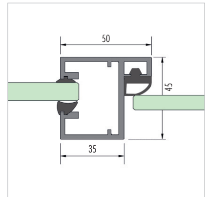
3 Zargenprofil, Anschluss Wandprofil
