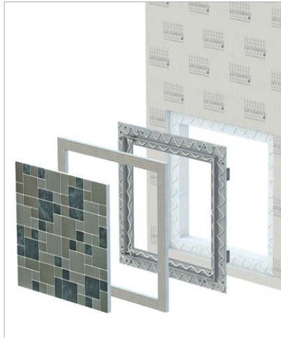
Anwendung bei Mosaikfliesen: mit Frontplatte / Füllstücke auf Rahmen
