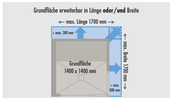
(Abbildung inkl. Blende)
